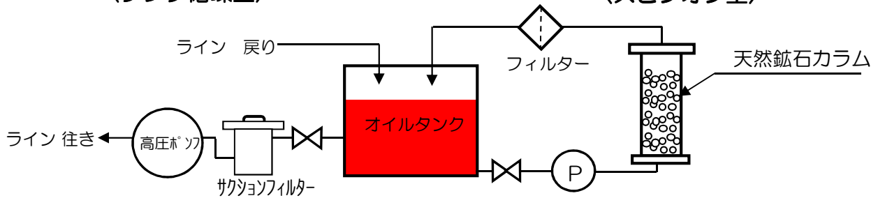
〈タンク循環型フロー図〉
